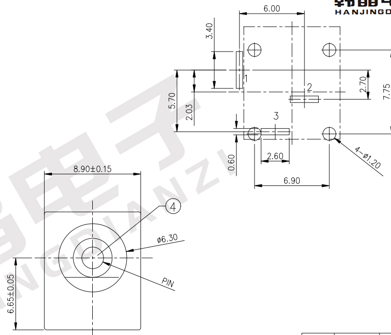
线路板开孔尺寸图
